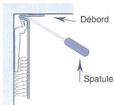
BOURRAGE DE LA BAVETTE OU DU DÉBORD
