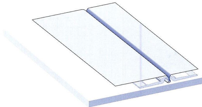
POSE RACCORD À PLAT «FAUSSE COUTURE»
