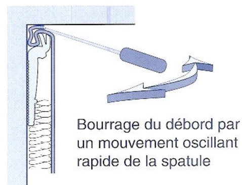
BOURRAGE DE LA BAVETTE OU DU DÉBORD
