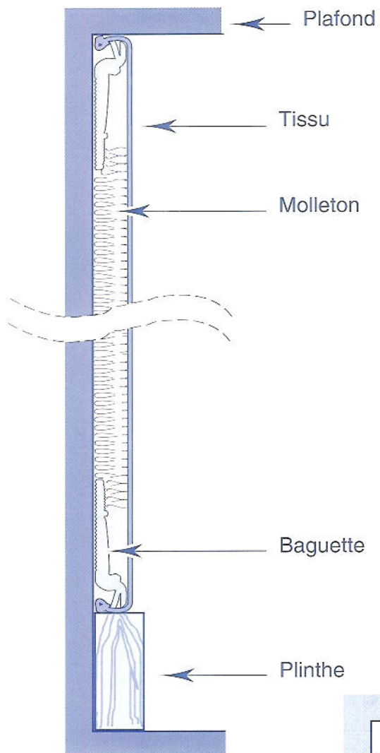
POSE ENTRE PLAFOND ET PLINTHE
